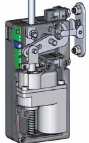
Elektromechanische Verriegelung
