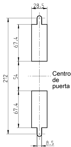
Corte
